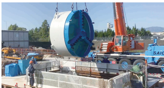
八王寺川バイパス管築造工事の様子
