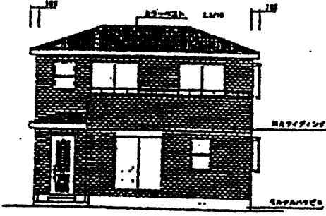
西立面図
