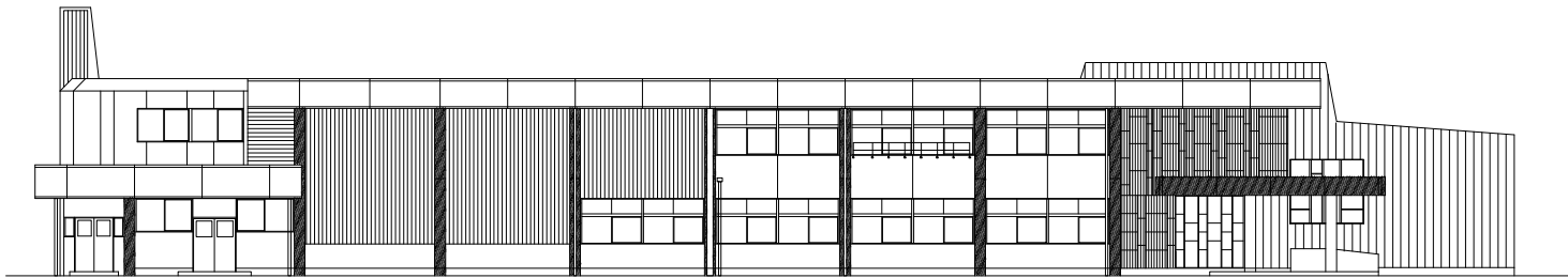
西 立面図
