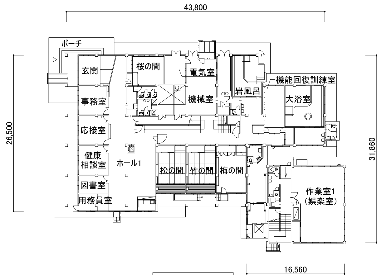
1階平面図
