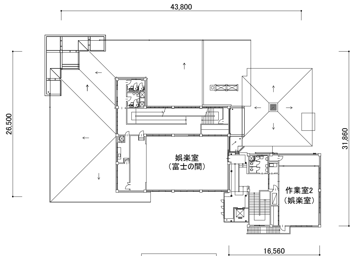
2階平面図
