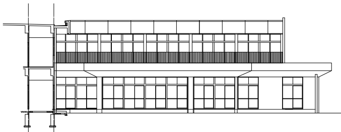
中庭南 立面図
