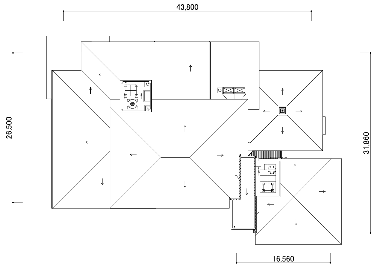
R階平面図
