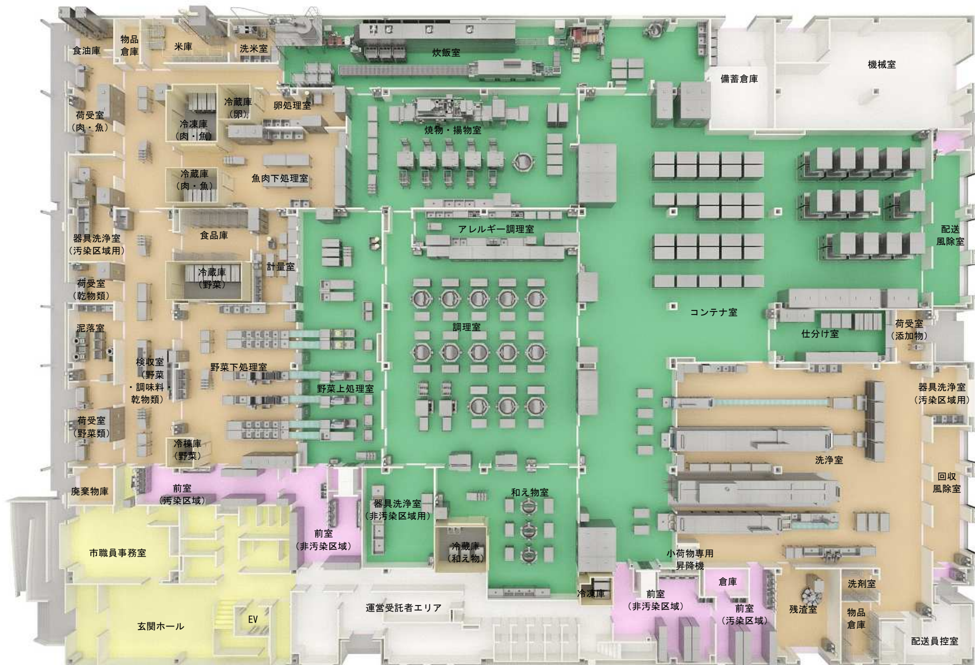
池田市立学校給食センター 調理場レイアウト図
