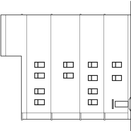
西側立面図
