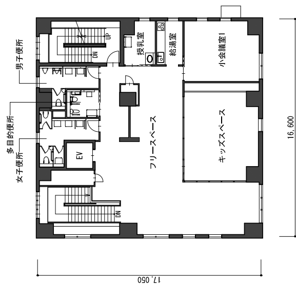
2階平面図
