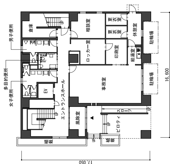
1階平面図
