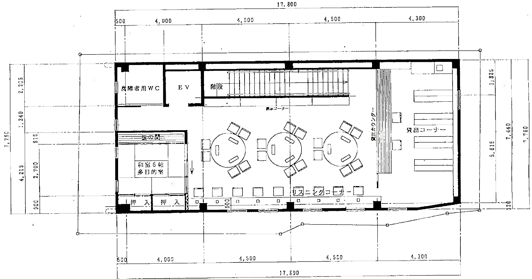
池田市立上方落語資料展示館 2階平面図
