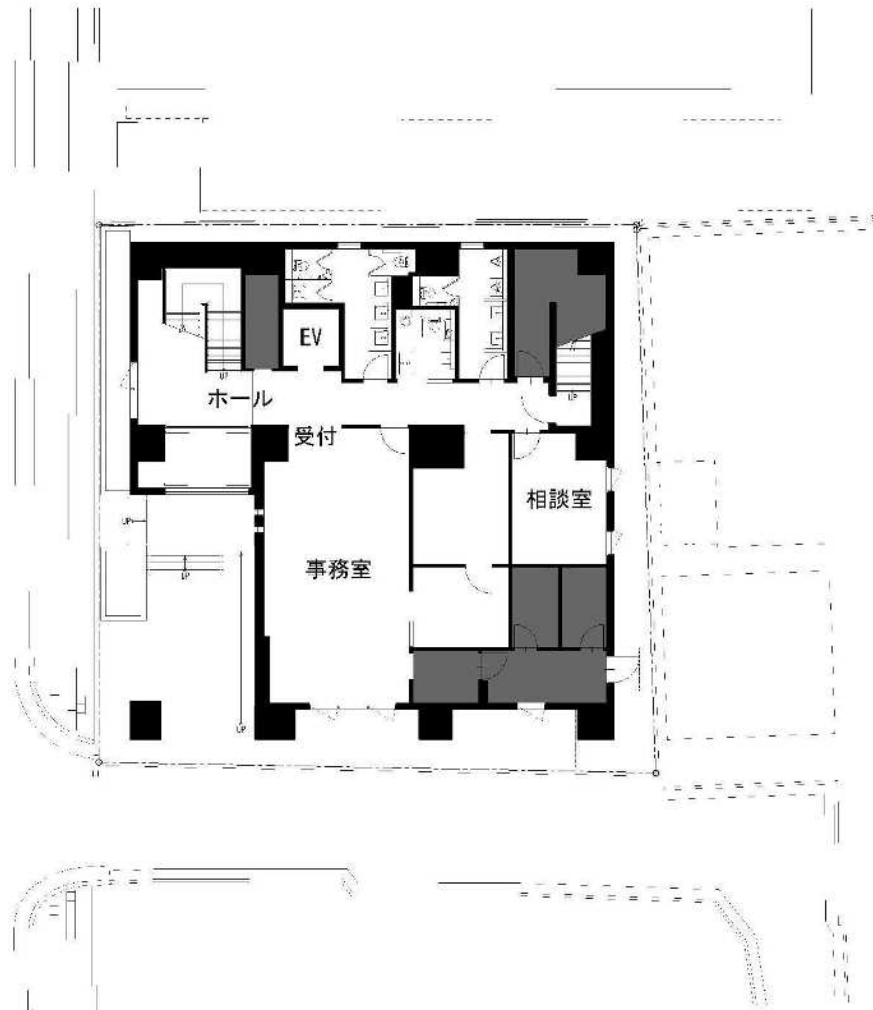
配置図兼1階平面図
